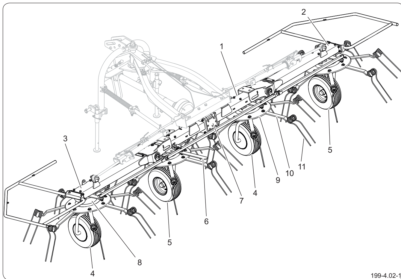
Рисунок 4.3 Конструкция модуля
