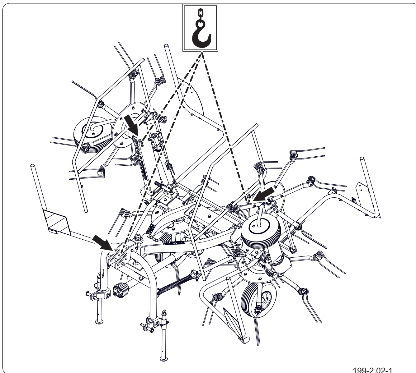
Рисунок 2.5 Точки крепления
