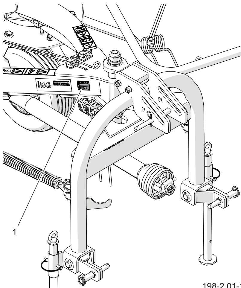
Рисунок 2.1 Идентификация машины
