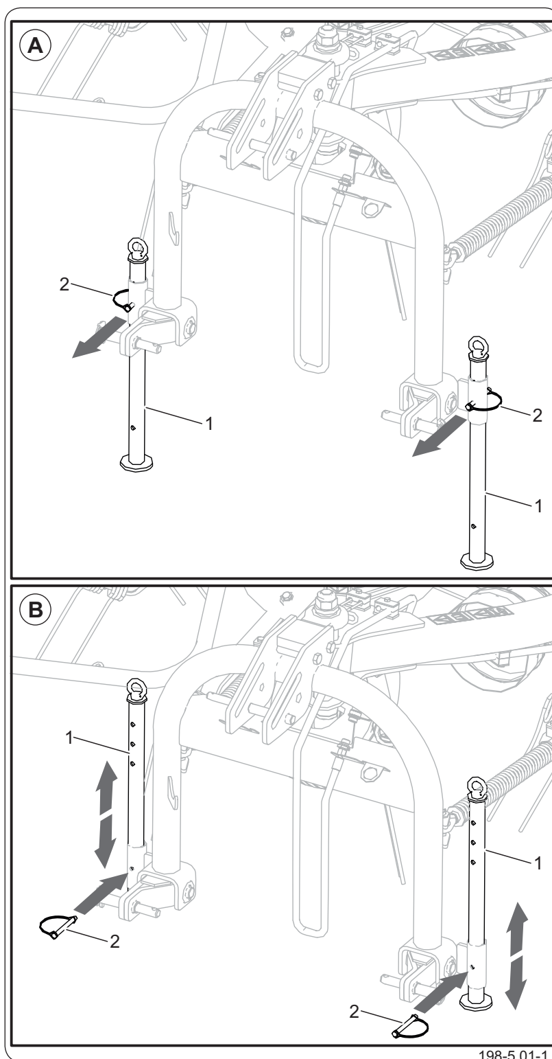
Рисунок 5.5 Стояночные опоры
